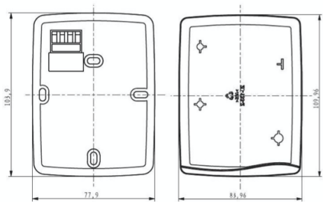
墙装型
