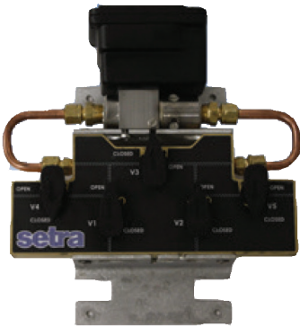
5 阀阀组
