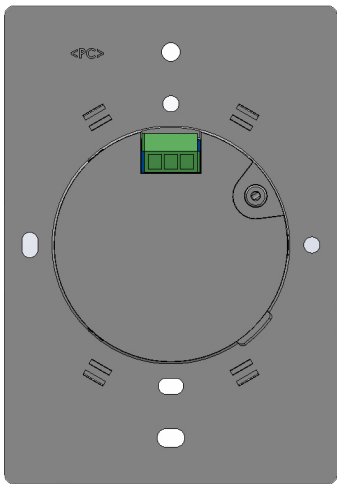
可见接线和压力接口的背视图
