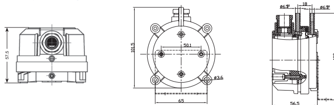
导压接管外形尺寸
